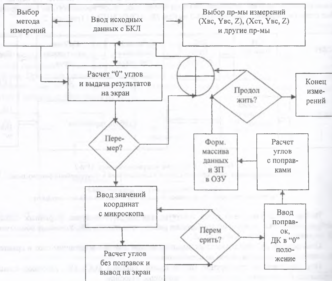
Рисунок 3 – Алгоритм измерений углов следов частиц в ядерных взаимодействиях
