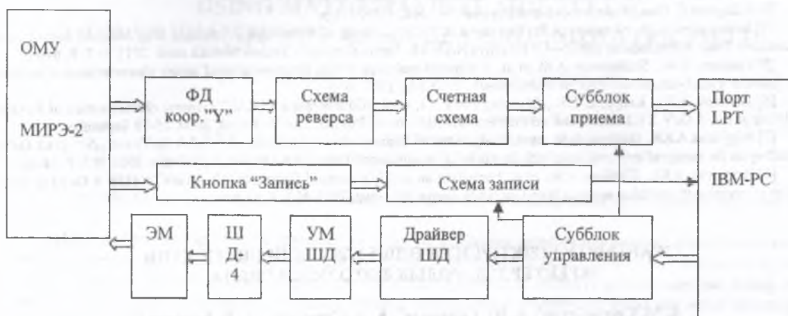
Рисунок 4 – Блок-схема модернизированного АРМ для измерения многократного кулоновского рассеяния заряженных частиц
